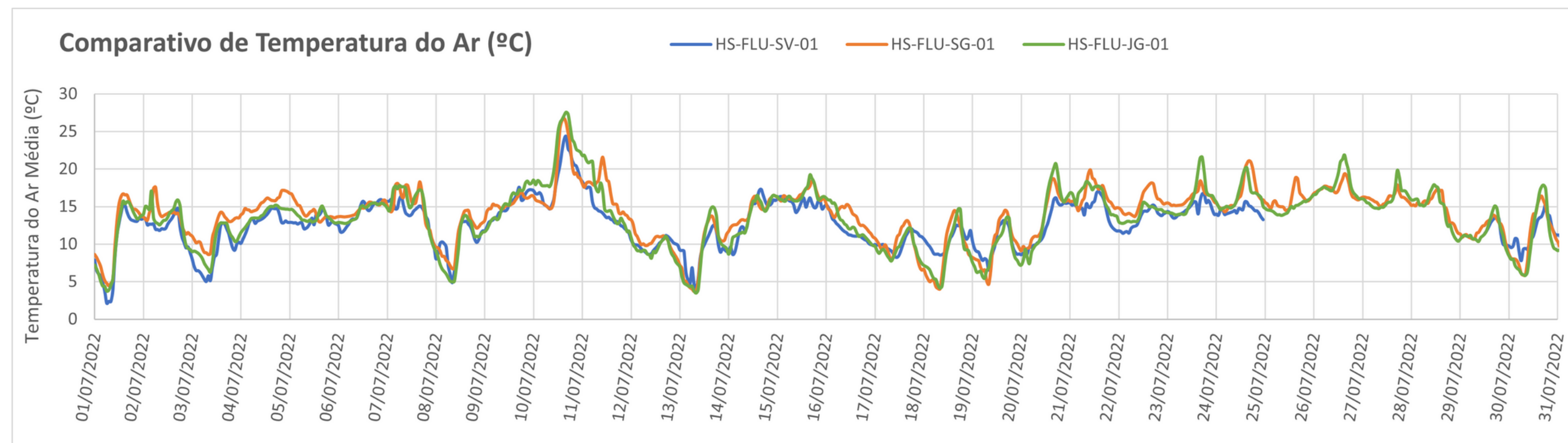
Figura 19 – Temperatura média do Ar (°C) comparativa nas Estações supracitadas:
